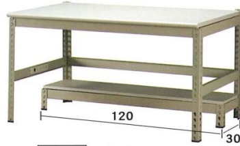
29002 工作桌 寬120x深70x高76(cm)
