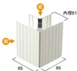
509 方外轉角組合
