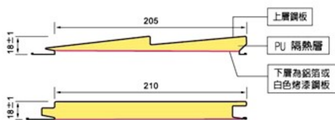
● 205型麒麟板斷面圖
