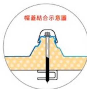
加上帽蓋(隱藏式)
