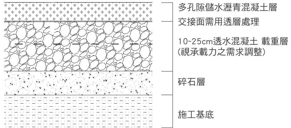
剖面示意圖
