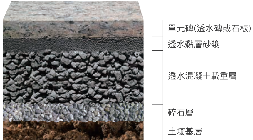
剖面示意圖
