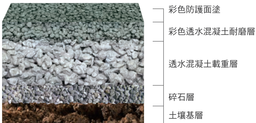
剖面示意圖
