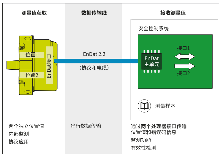
带EnDat 2.2的高安全性位置编码器
