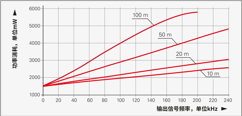
HTLs接口的功率消耗（最大）和供电电压U P = 30 V
