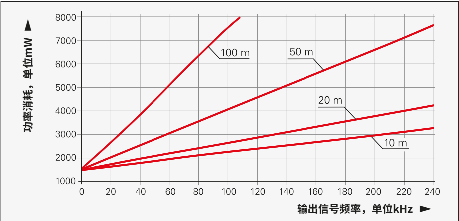
HTL接口的功率消耗（最大）和供电电压U P = 30 V
