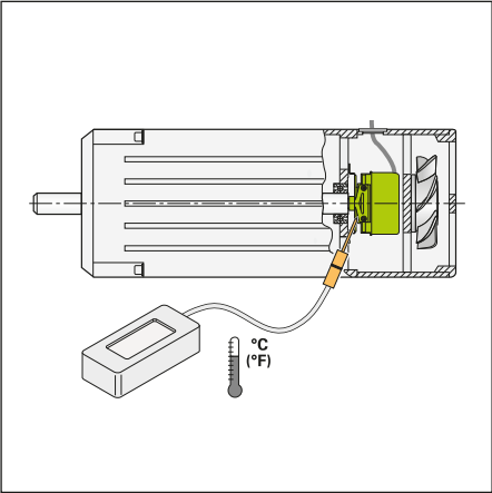
在旋转编码器的指定位置处测量实际工作温度（参见技术参数）
