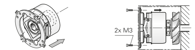
ECN/EQN/ERN 400带万能定子联轴器
