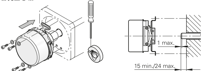
ECN/EQN/ERN 400带标准定子联轴器
