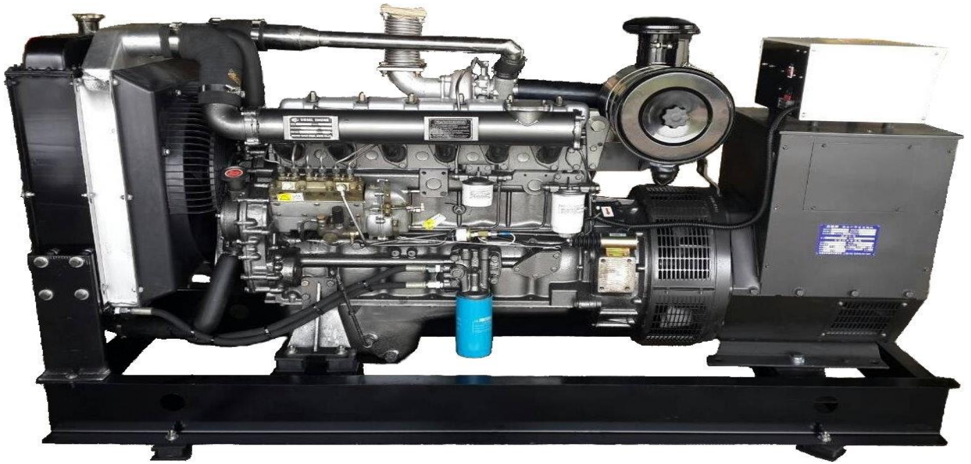
柴油引擎發電機組參考規格 《規格為參考值，資料如有變更恕不另行通》
