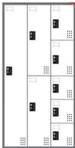
FC1-3 系列 寬=90cm / 高=180cm 900W x 510D x 1800H mm
