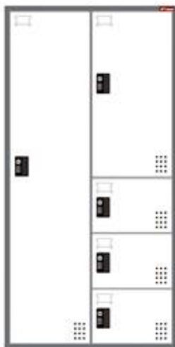
FC1-2 系列 寬=90cm / 高=180cm 900W x 510D x 1800H mm
