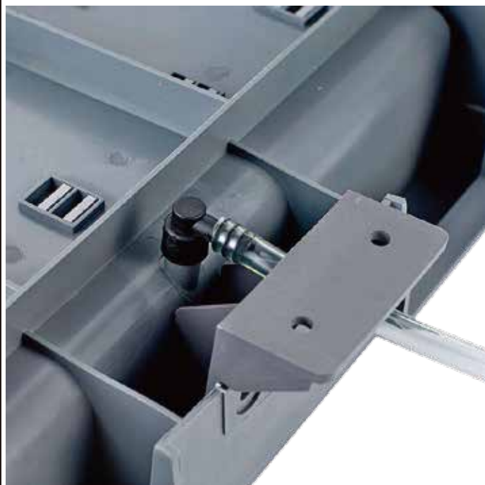
排水接管
