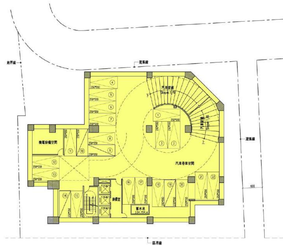
地下肆層平面圖
