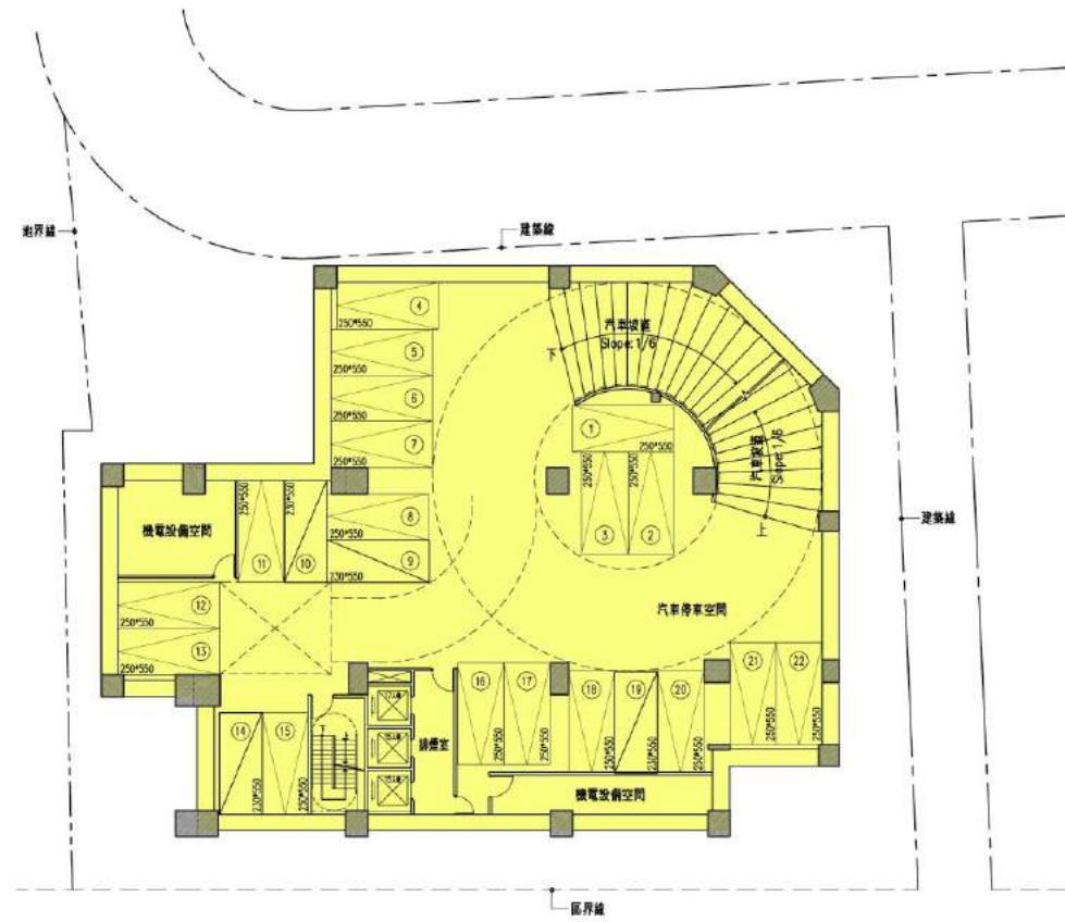
地下貳至參層平面圖
