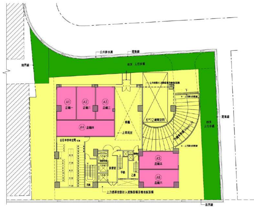
壹層平面圖
