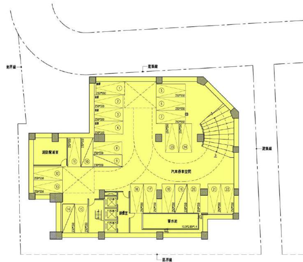
地下伍層平面圖
