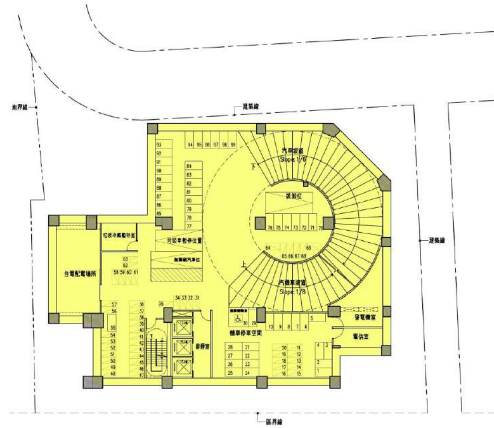
地下壹層平面圖
