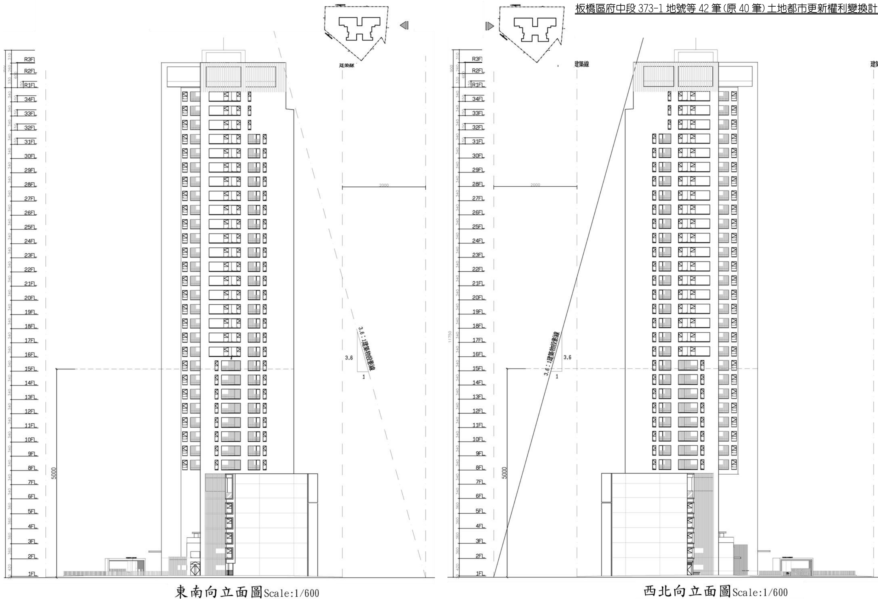
圖 6-25 東南向及西北向立面圖 S:1/600
