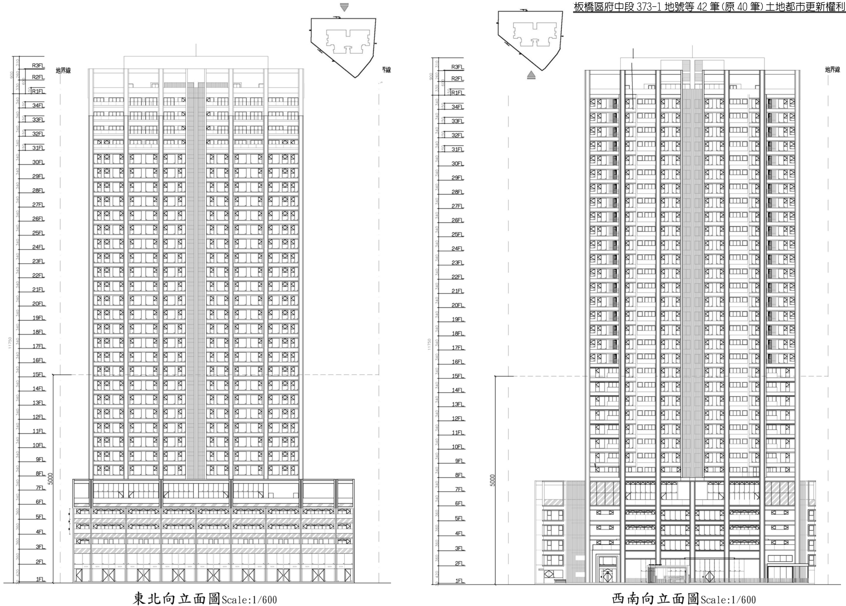
圖 6-24 東北向、西南向立面圖 S:1/600
