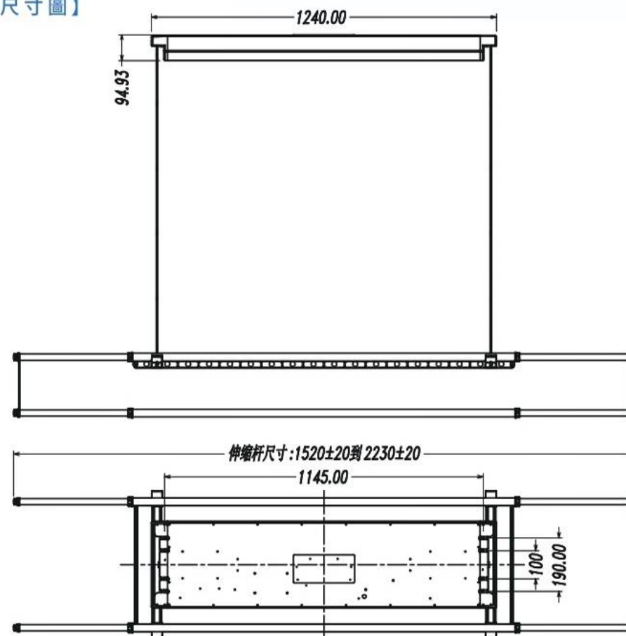
【尺寸圖】
