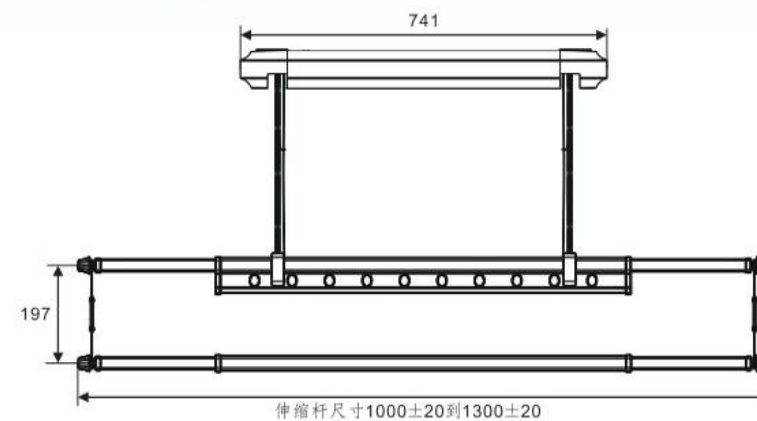
【尺寸圖】
