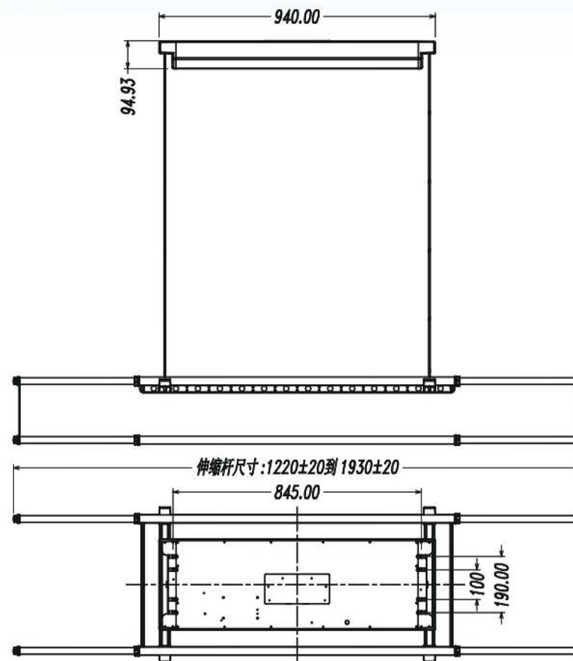
【尺寸圖】
