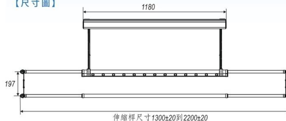
【尺寸圖】
