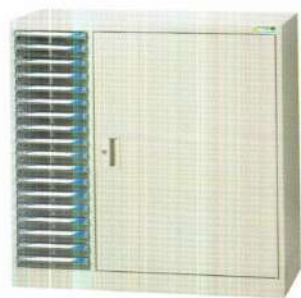
43007 3尺A4單開門18小抽 寬88x深41.5x高88(cm)
