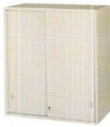
3-15 鐵拉門上置式鋼製公文櫃 W900xD450xH1062(mm) NT $ 2550 ◆訂購數量限1組(含)以上, 200組(含)以下
