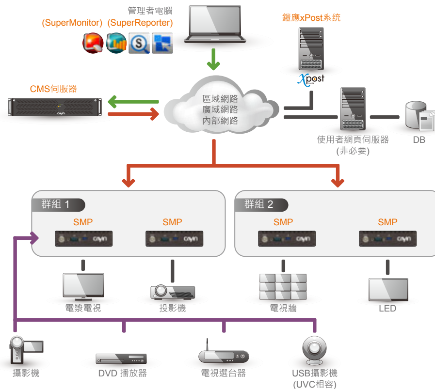
主從架構下的數位看板網絡 (CMS伺服器 + SMP數位看板播放器)
